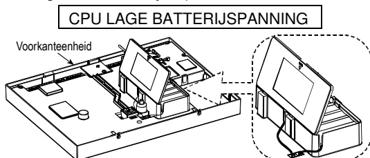
Figuur 10. Batterijvervanging
